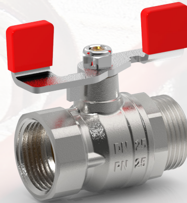
DN15-DN32 PN25
